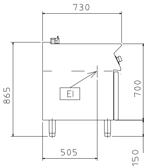
Zij aanzicht
